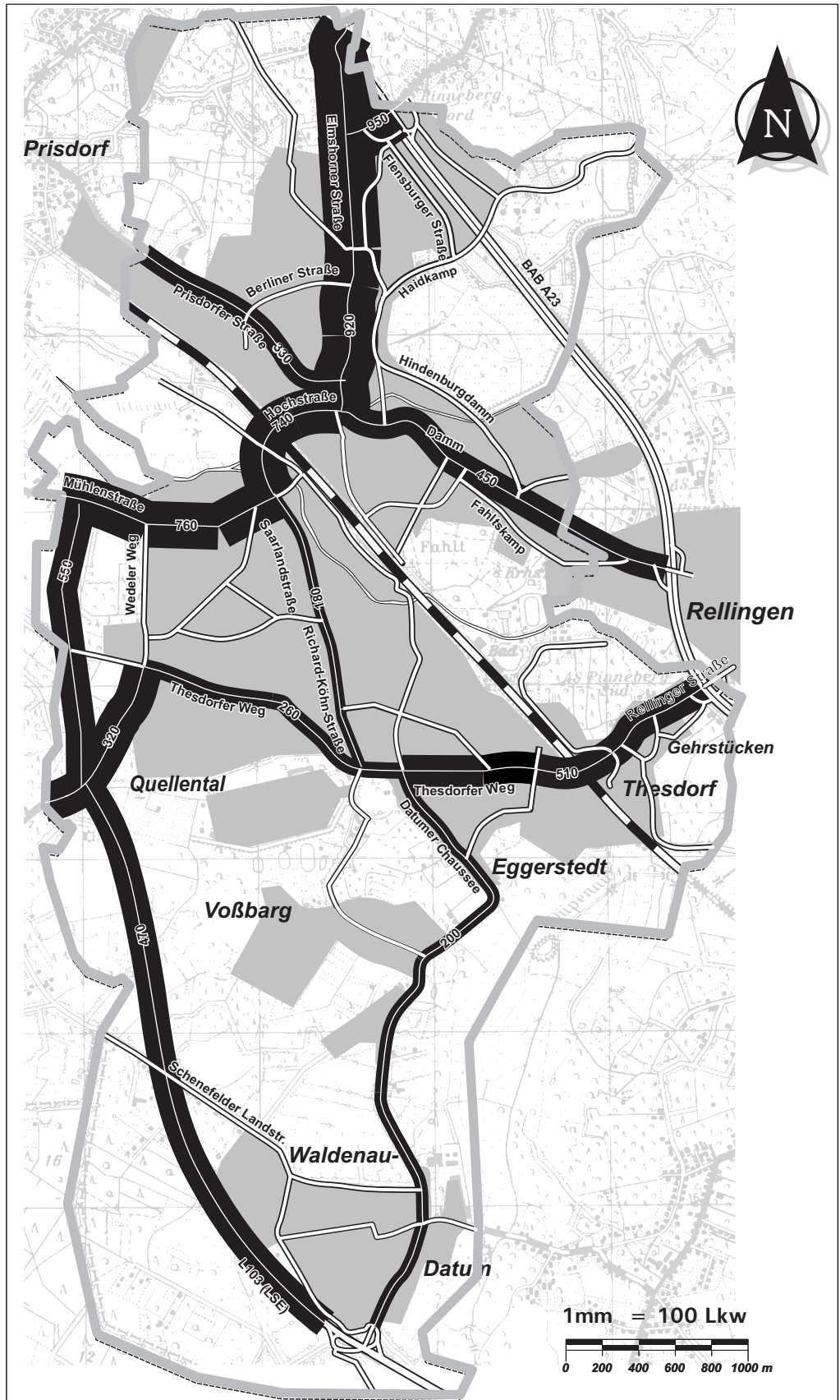
2: Verkehrsbelastungen [Lkw/24h] Querschnittszählung 2006
