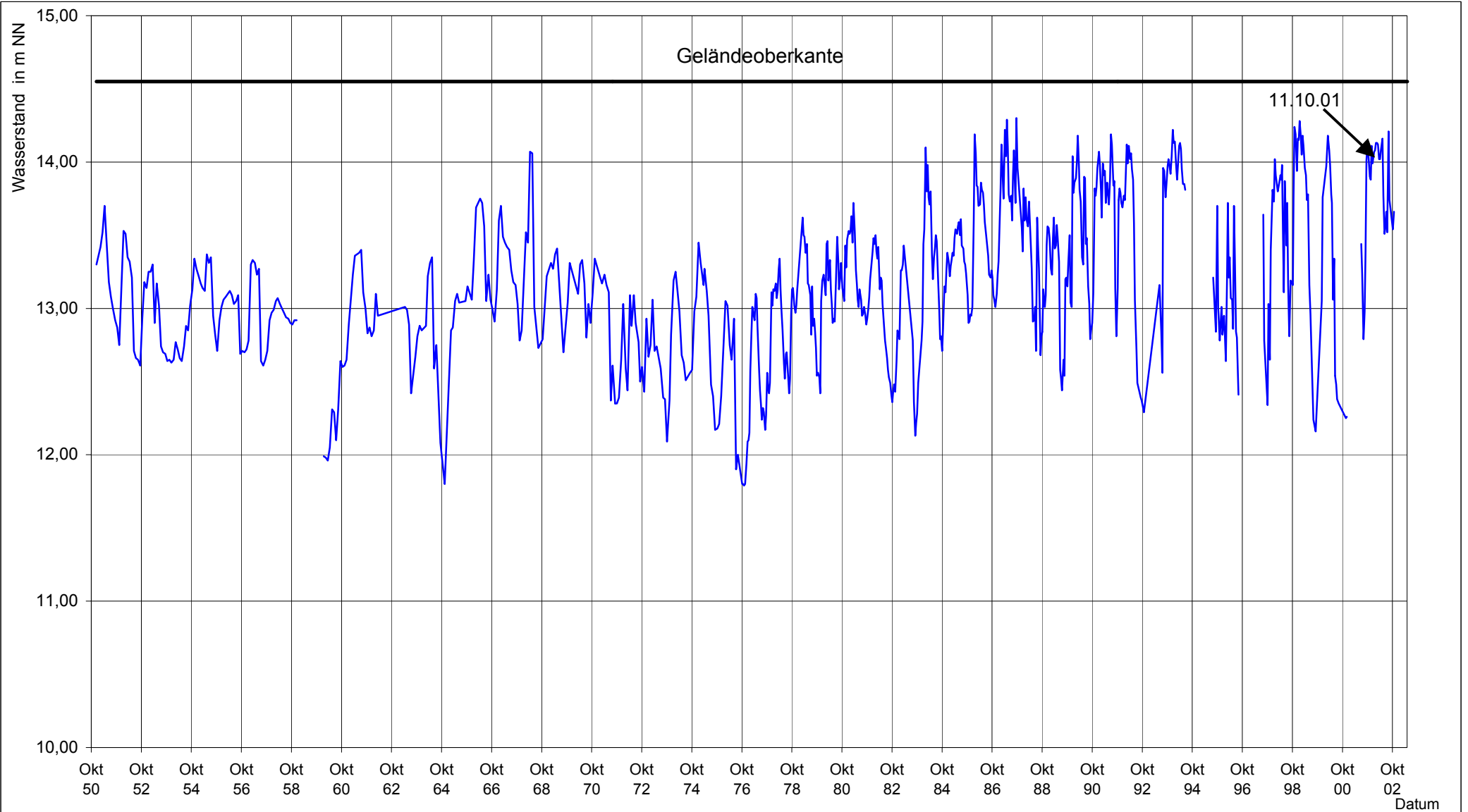
Anl. 6: Grundwasserstandsganglinie der Grundwassermessstelle 53, Zeitraum 01.10.1950 bis 30.04.2003
